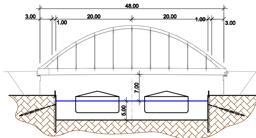
KOMBINOVANÝ PROFIL
